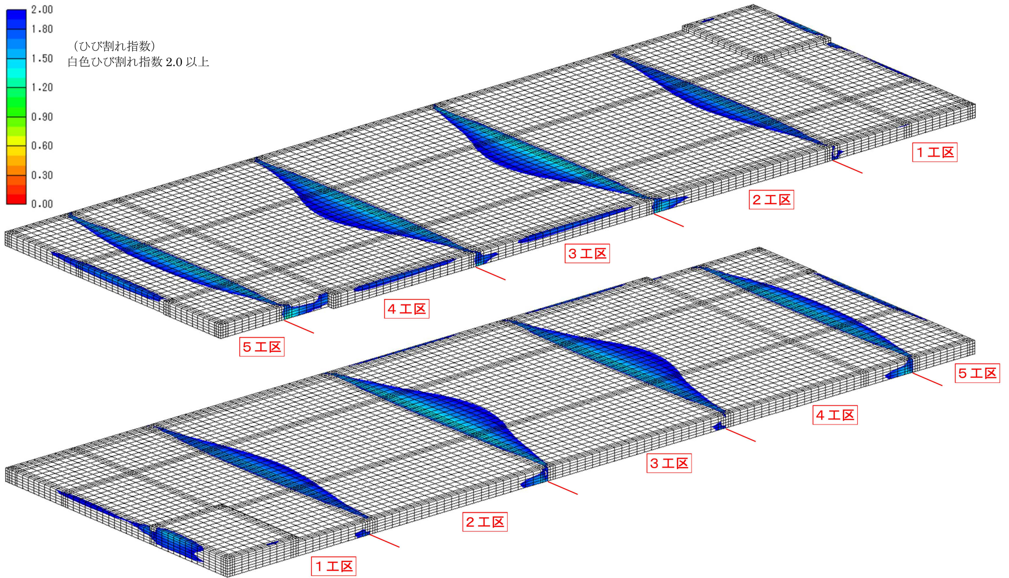
図4 耐圧版表面ひび割れ指数の分布図
